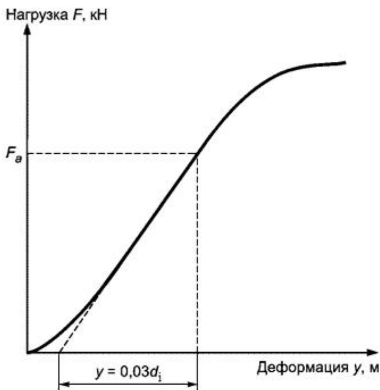
Рисунок В.1 - Кривая "нагрузка-деформация"
